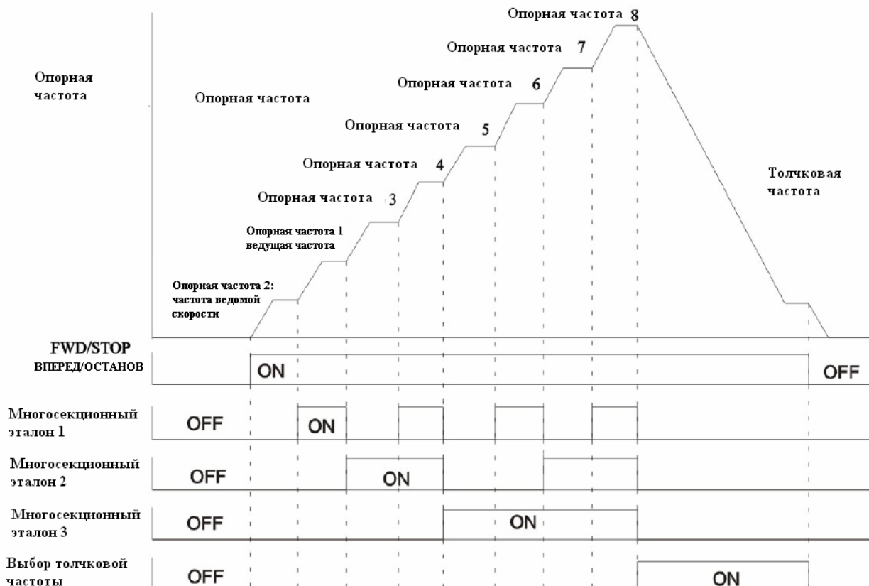
Схема последовательности сигналов многосекционного эталона/ выбора толчковой частоты
