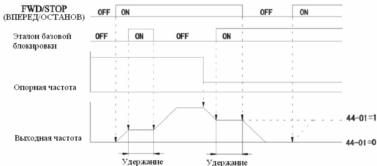
Ускоренный и замедленный останов
