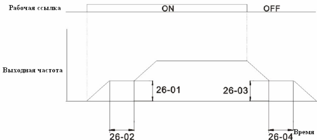
Схема последовательности операций функции DWELL (Задержки)
